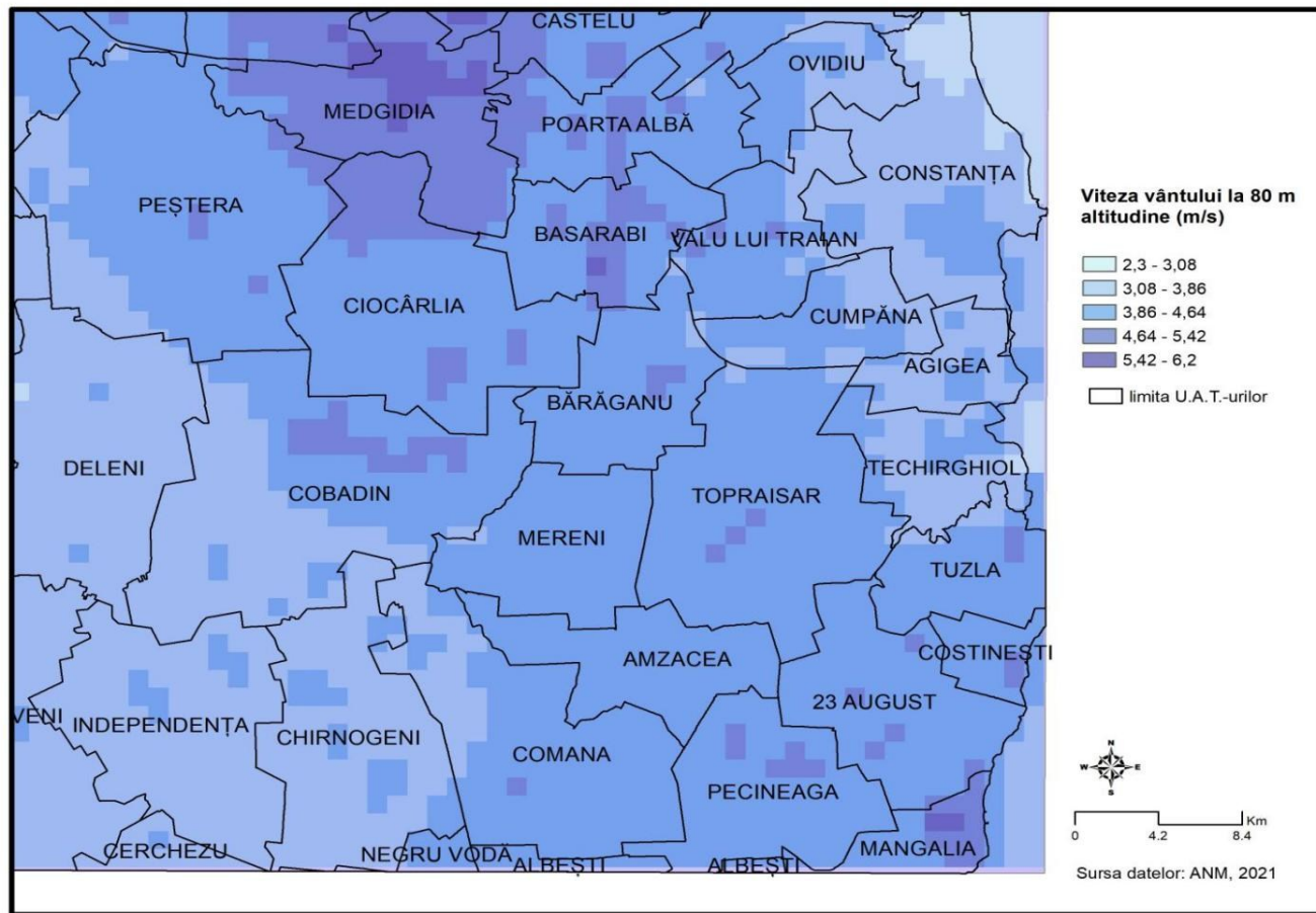
Figura 1.4. Potențialul eolian al Dobrogei de Sud, pe baza vitezei medii a vântului
