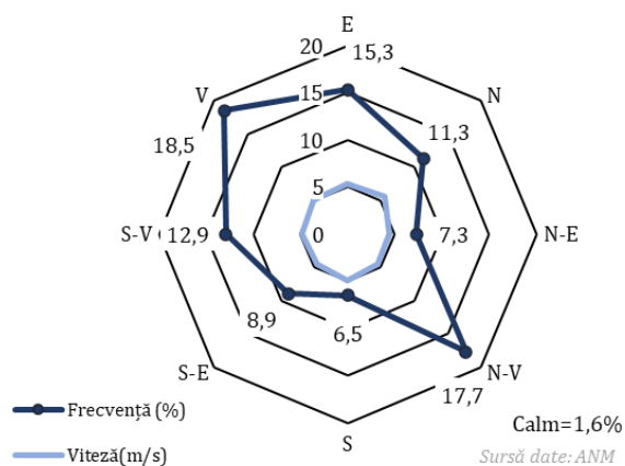
Frecvența și viteză medie lunară a vântului pe 8 direcții, înregistrate în luna decembrie 2021, la stația meteorologică Medgidia
