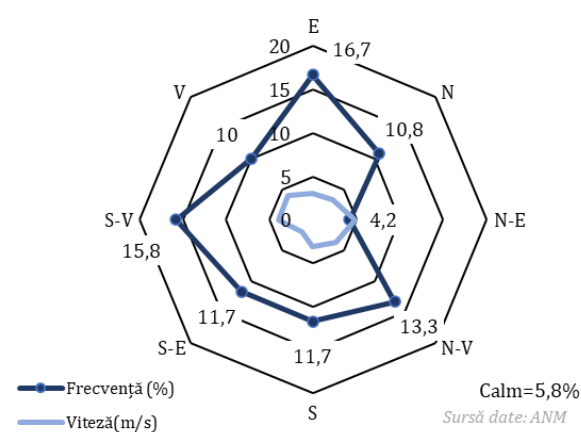
Figura 1.3. Frecvența și viteză medie lunară a vântului pe 8 direcții în municipiul Medgidia în 4 luni ale anului diferite
